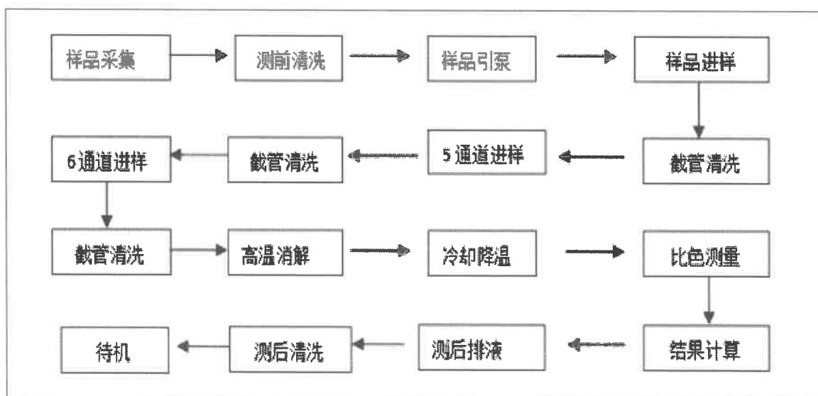
测量流程图
