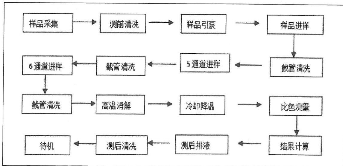
测量流程图
